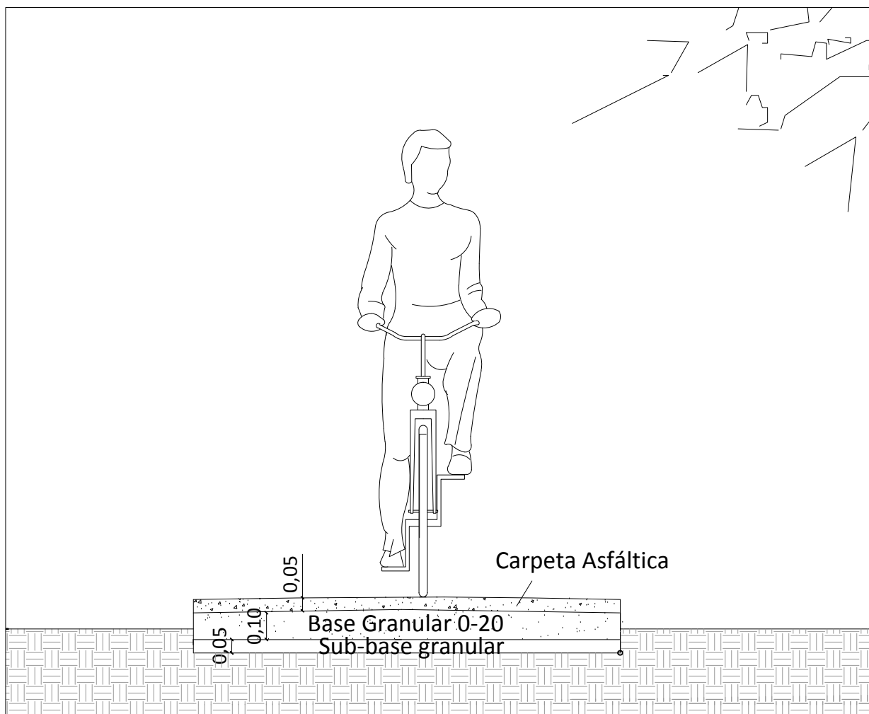
DETALLE CICLOVÍA - Esc. 1:25
